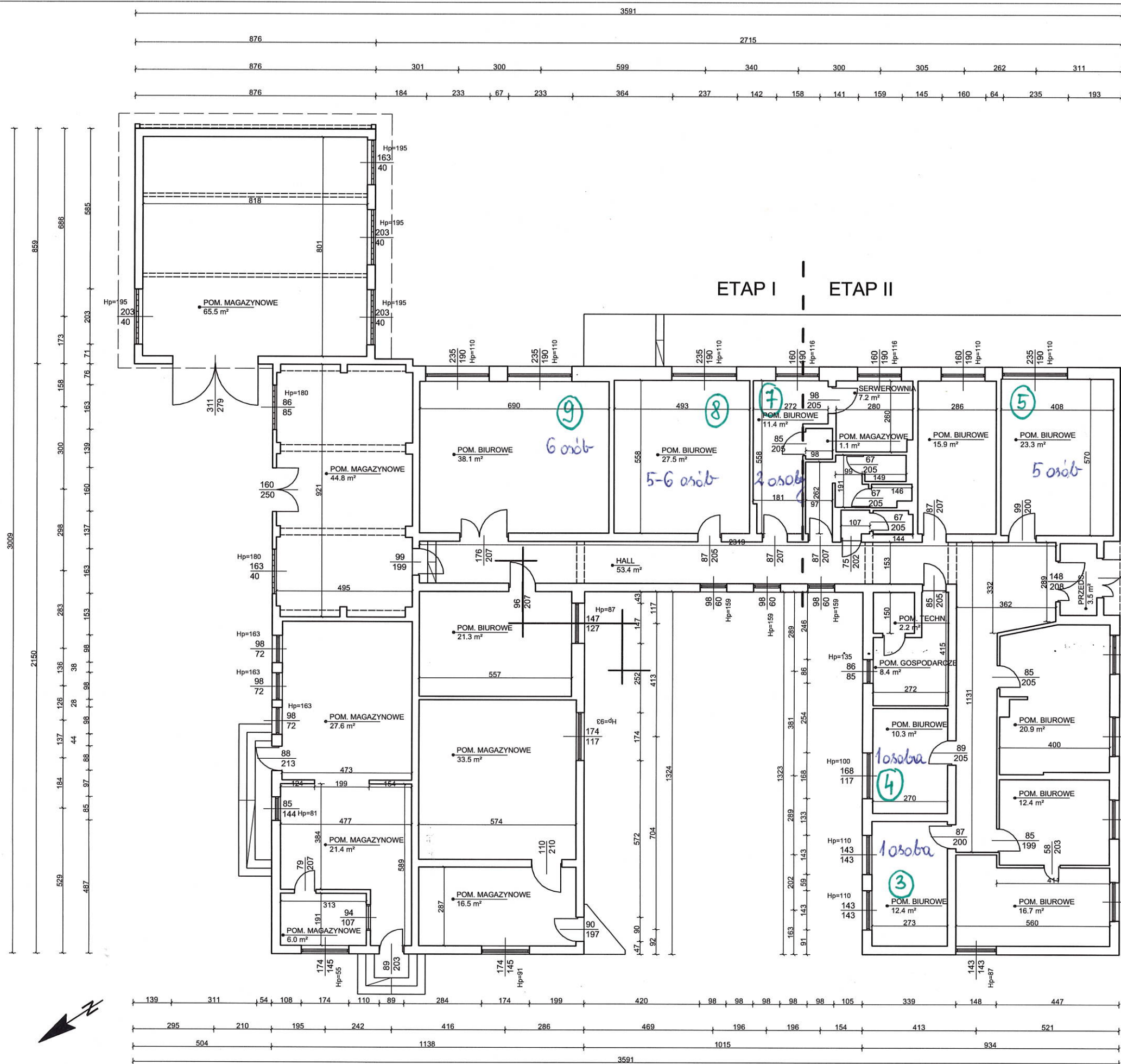
RZUT PARTERU SKALA 1:100
